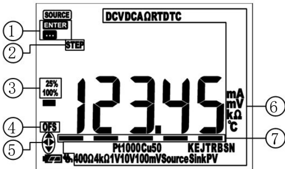
图 5.1 常规操作状态显示画面
