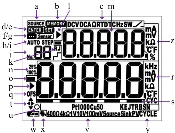
图 3.2 显示屏示意图
