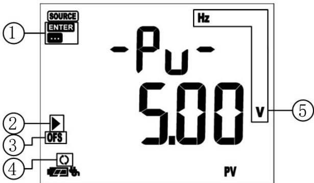
图 5.5 频率类型信号操作时的显示画面 2：脉冲幅值修改
