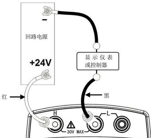
图 5.2 模拟变送器模式的接线方式
