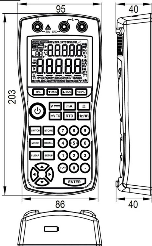
图 3.1 外形尺寸图 (单位: mm)
