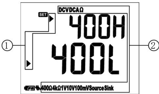
图 5.11 校准参数菜单状态
