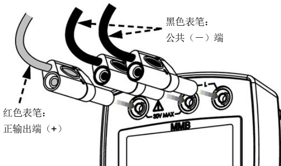
图 3.5 表笔接口示意图
