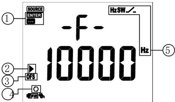
图 5.4 频率类型信号操作时的显示画面 1：频率值修改
