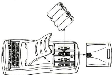
图 4.1 电池安装示意图
