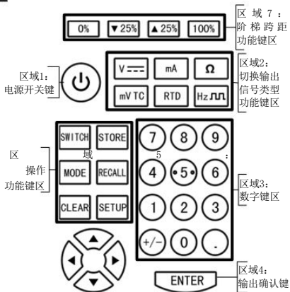
图 3.3 按键区示意图
