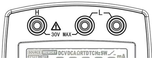
图 3.4 输出端子示意图
