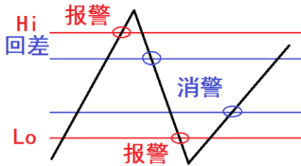
图 4-1 高低报警及回差的图例
