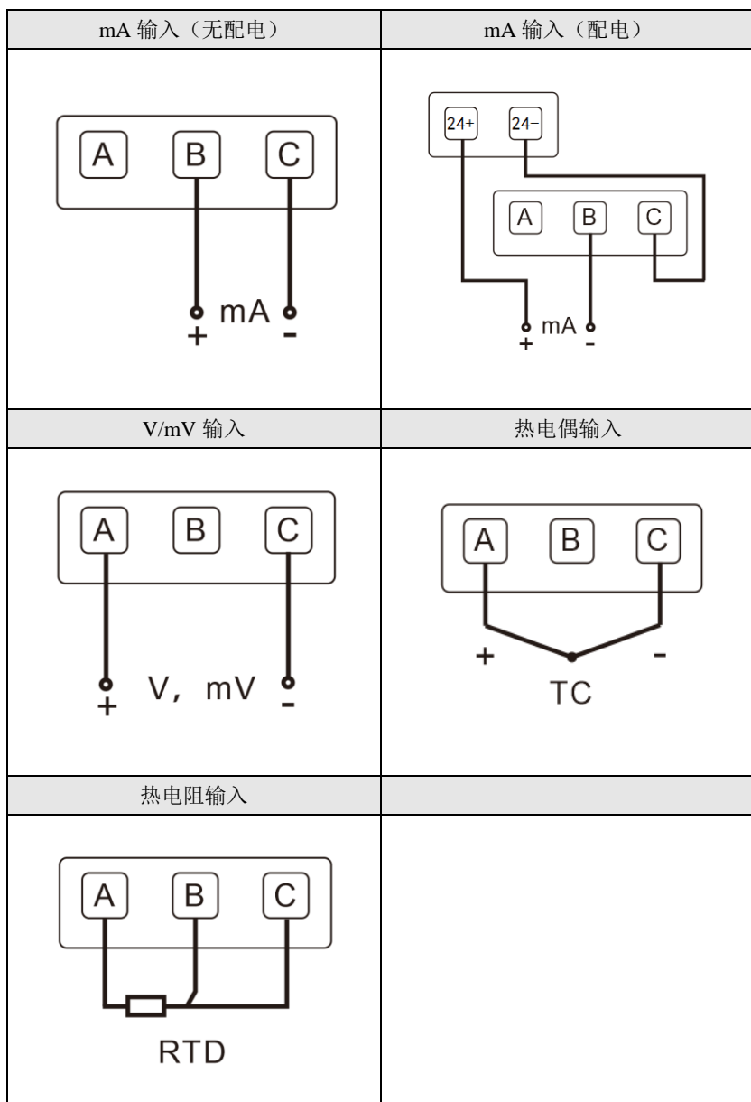
图 2-4 信号线连接示意图
