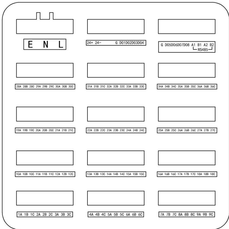
图 2-3 端子视图
