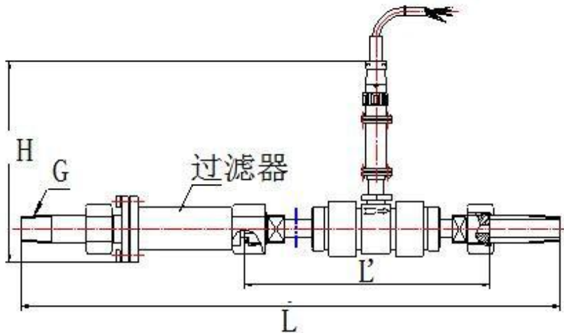
图 2 DN4~DN10 螺纹连接流量传感器结构及安装尺寸示意图
