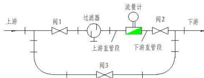
图 11 流量计安装示意图
