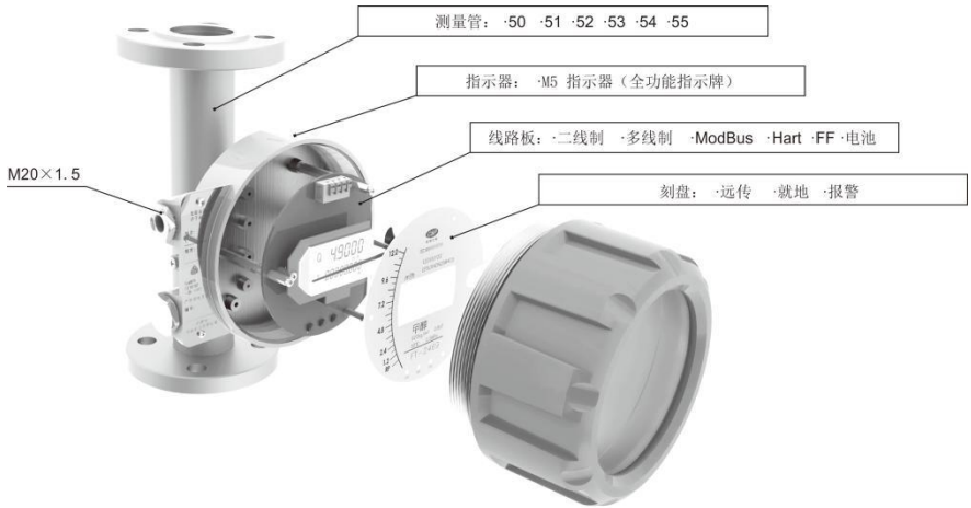
图 2 M5 指示器
