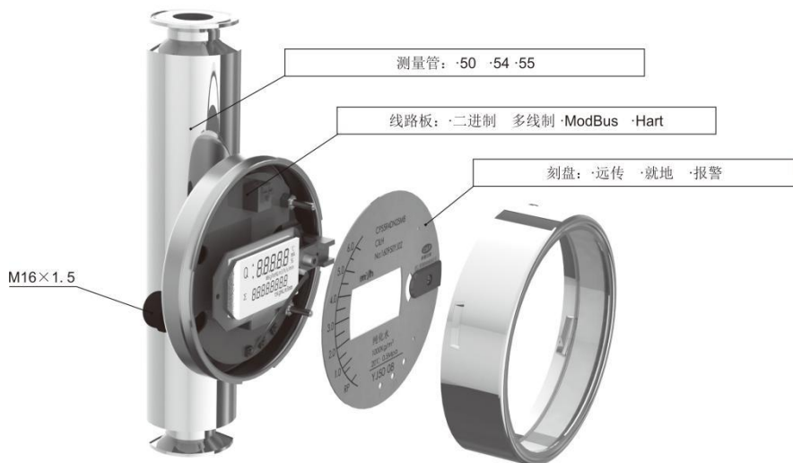
图 5 M8 指示器卫生型
